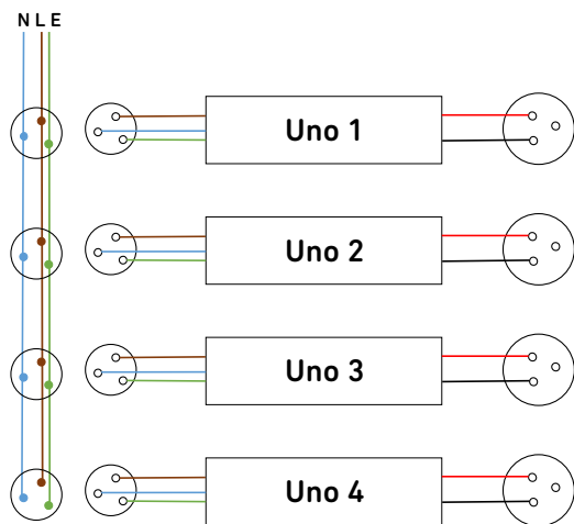
1 x 4 Elektroinstallasjon
