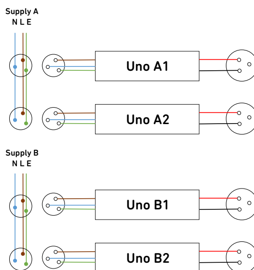
2 x 2 Elektroinstallasjon
