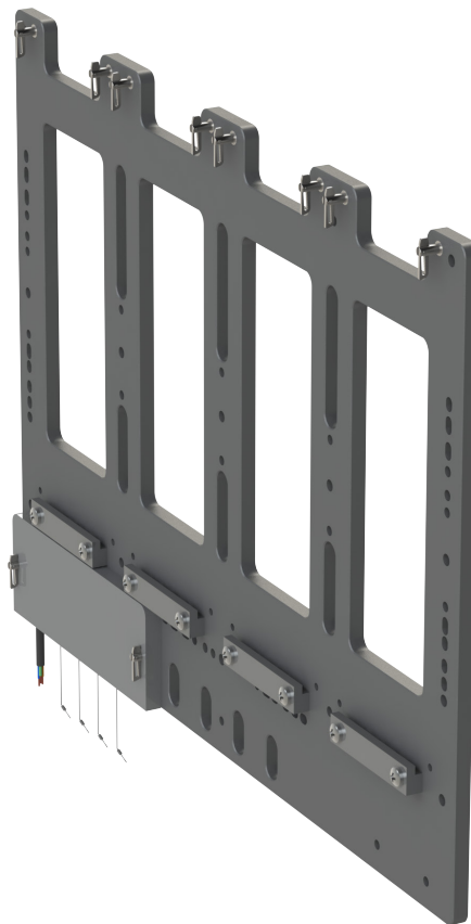
Klemmer og brakettesett som passer til ethvert havmerddesign
