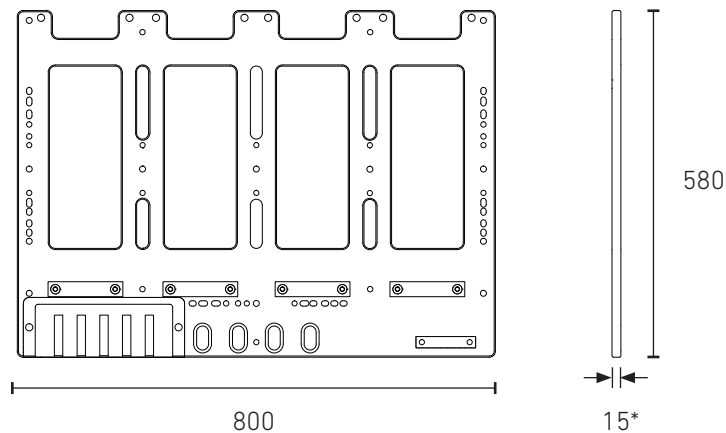
Uno Panel dimensjoner. Alle mål i millimeter (mm)
