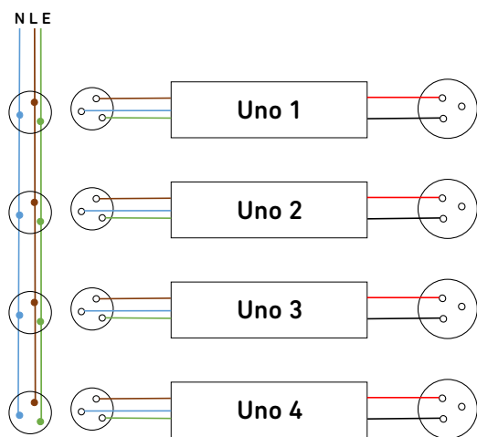
1 x 4 Elektroinstallasjon
