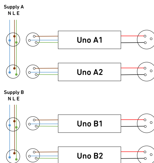
2 x 2 Elektroinstallasjon
