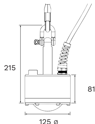
Fokus 600 dimensjoner Alle mål i millimeter (mm)
